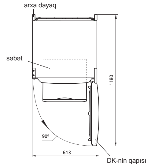
Şəkil 2 — Soyuducu (yuxarıdan görünüş)
